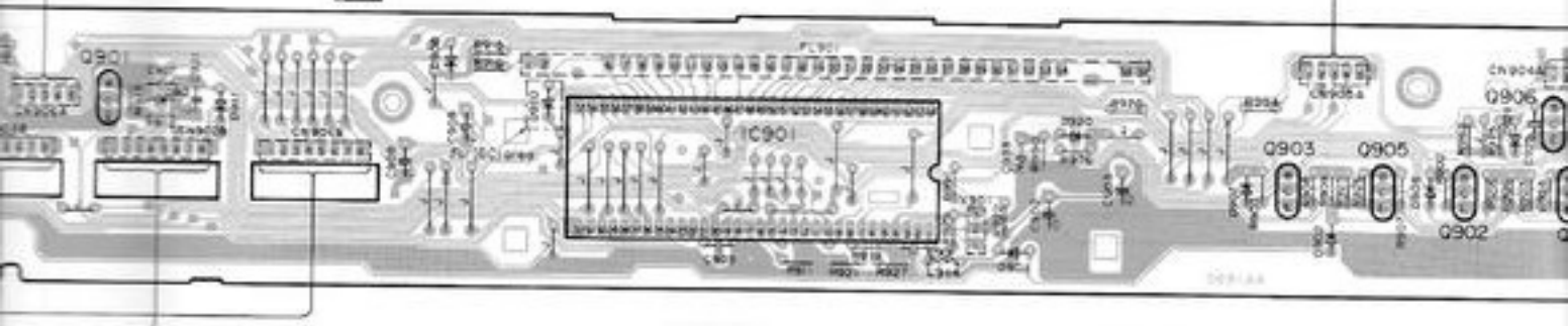
D FL DRIVE P.C.B.
