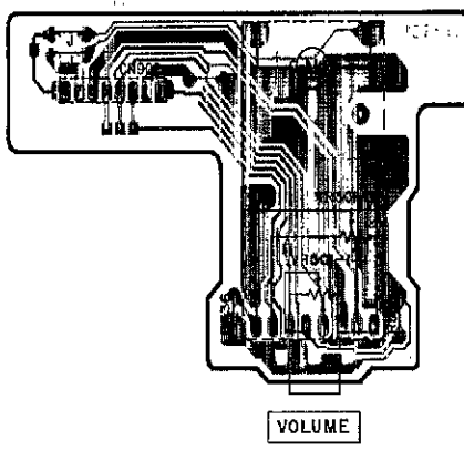
B VOLUME P.C.B. (REP1874A-S)
