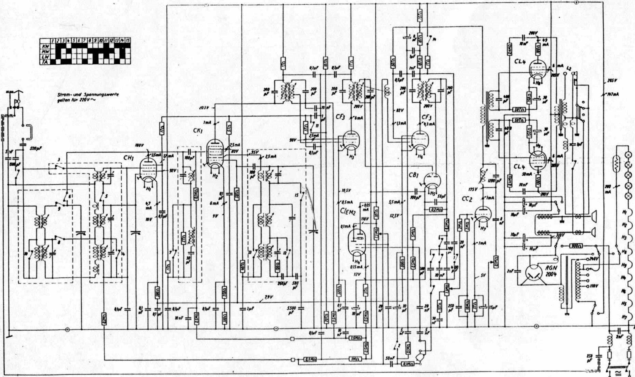
AEG, 97 GWK, und Telefunken, 7000 GWK, Allstrom, 2 Vorkreise, 6 Zwischenfrequenzkreise.
