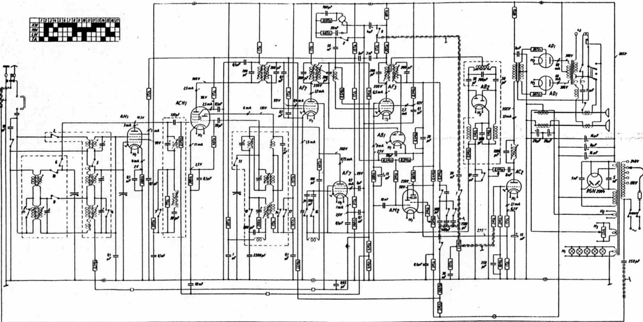
AEG, 107 W, und Telefunken, 7001 WK, Wechselstrom, 2 Vorkreise, 7 Zwischenfrequenzkreise.
