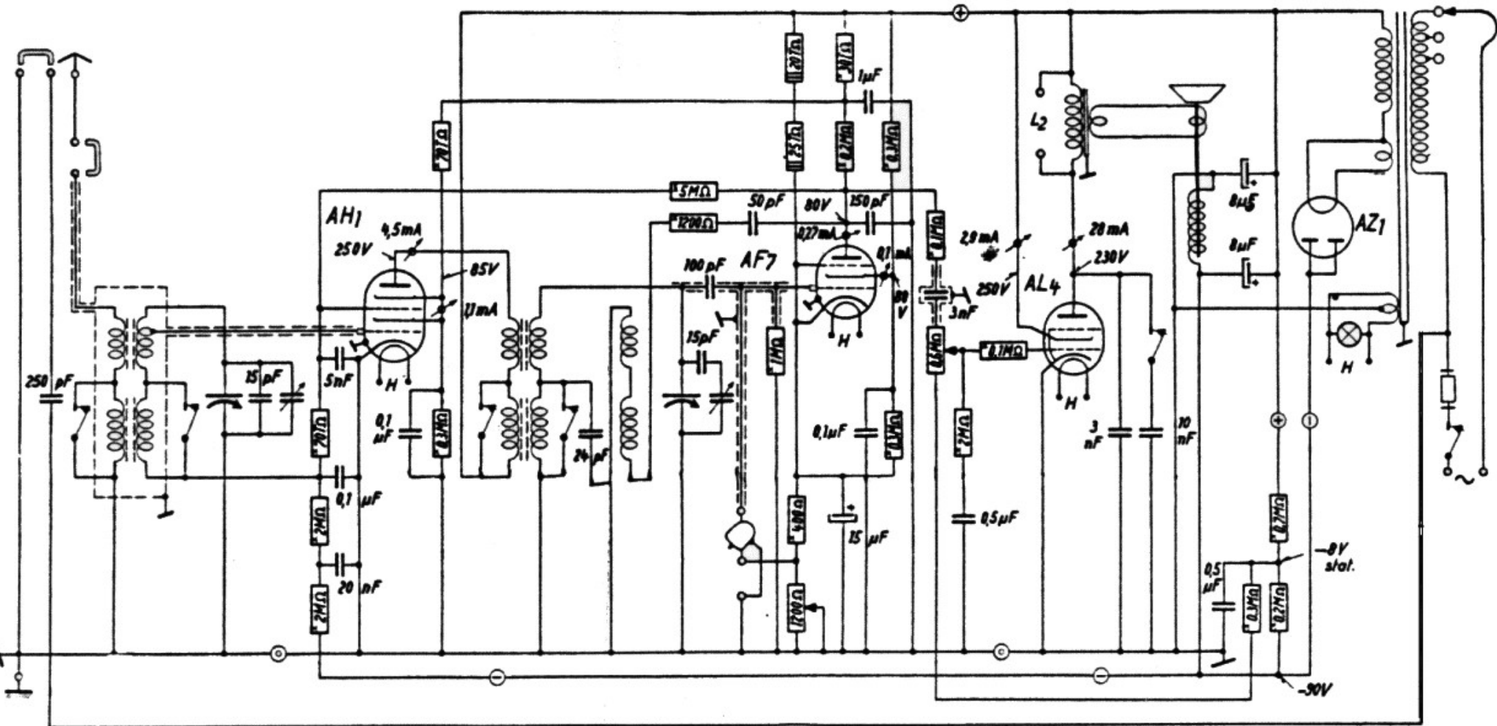
AEG, 27 W, und Telefunken 724W, Wechselstrom, 2 Kreise
