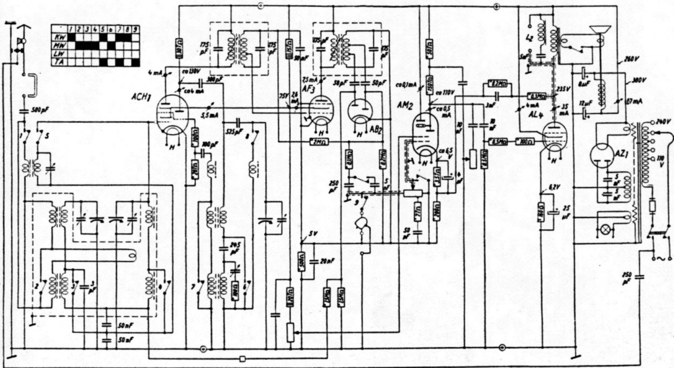
Telefunken, 776 WK, und AEG, 77 WK, Wechselstrom, 2 Vorkreise, 4 Zwischenfrequenzkreise
