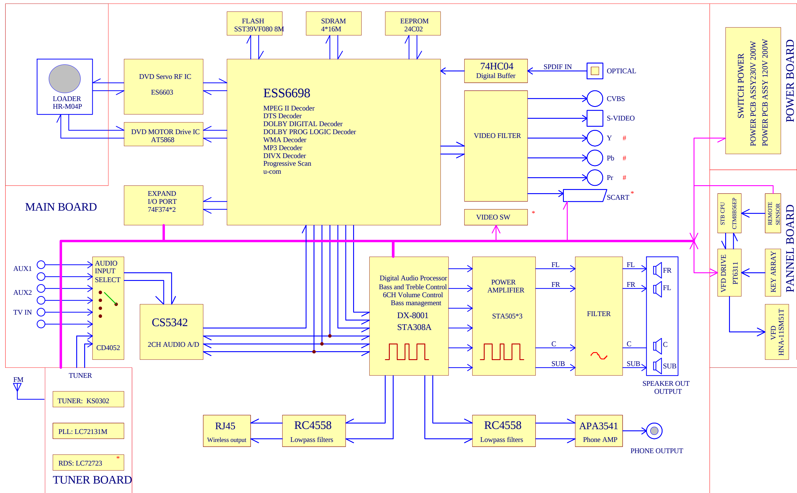
DPL930 / DPL2930 / RTD218 Block Diagram
