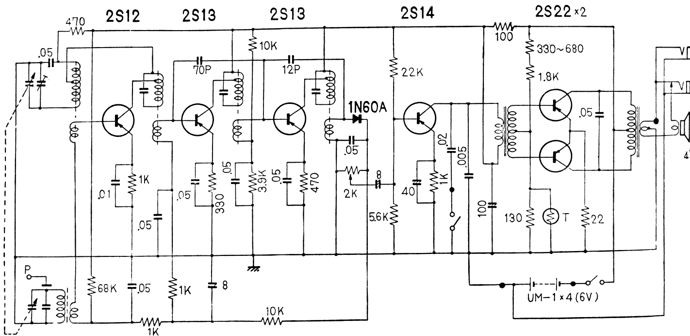
TOSHIBA 6TR-196, 200.
