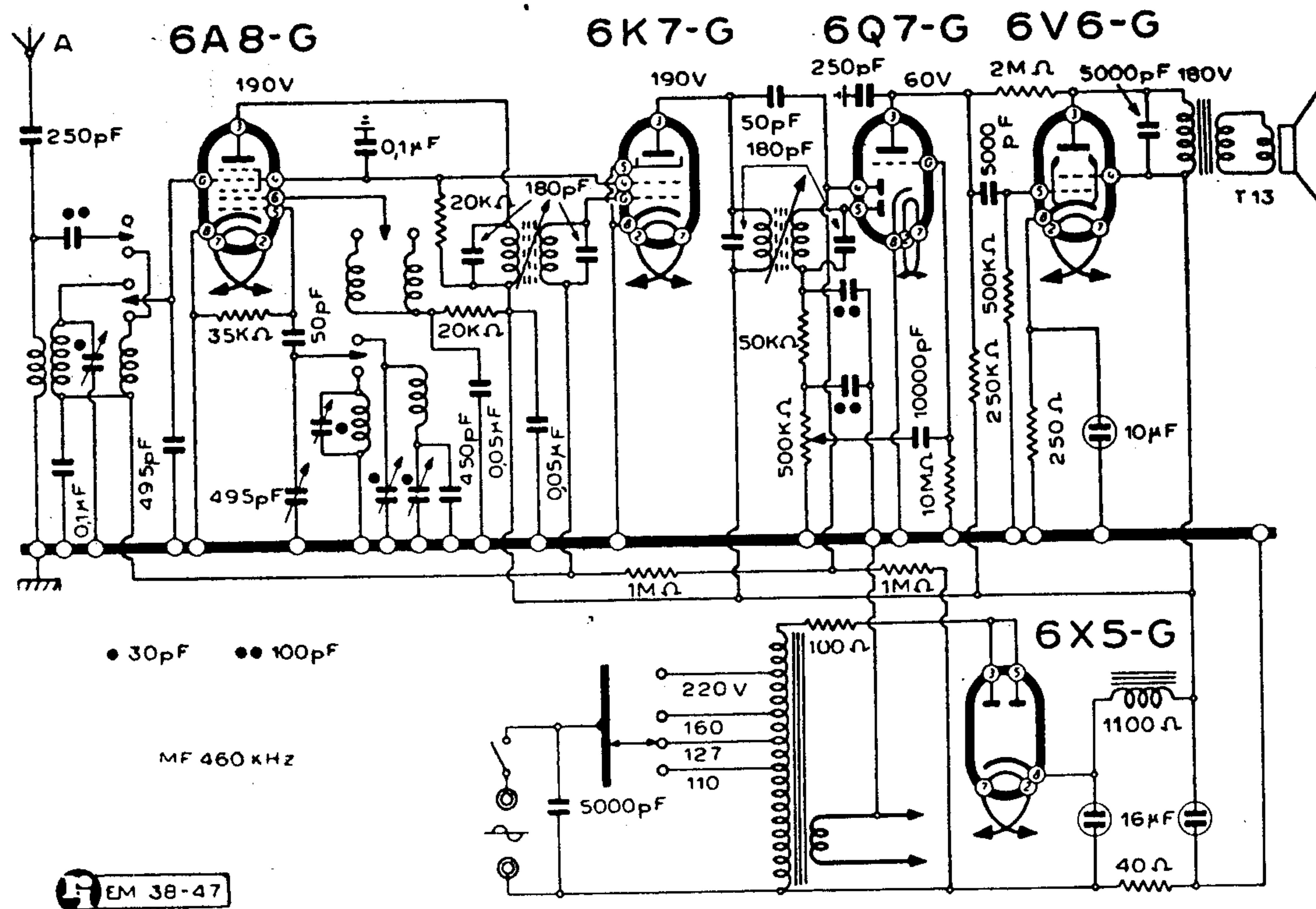
WATT RADIO - MOD. «AUREA PICCOLO» 1948
