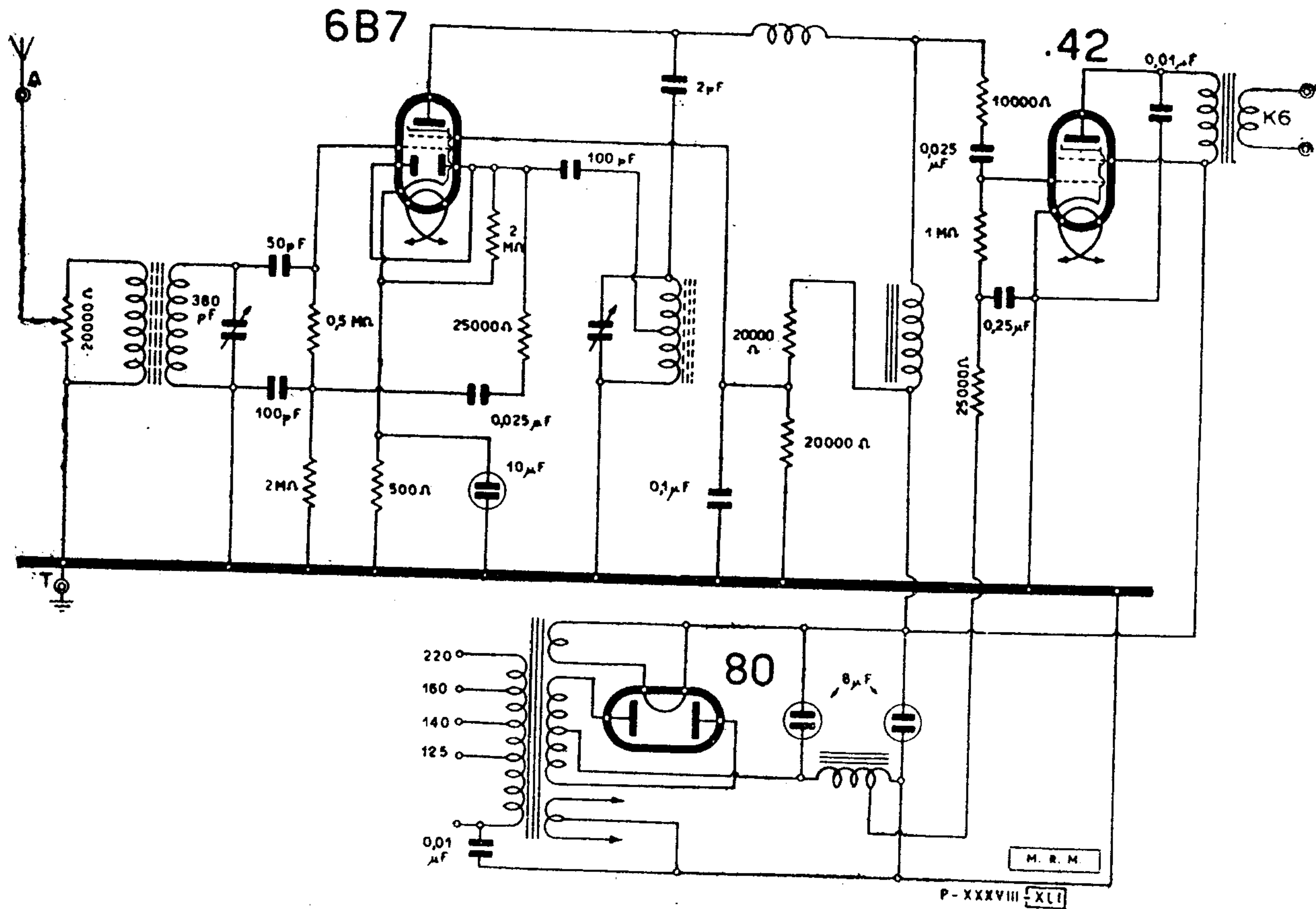
WATT RADIO - MOD. «BALILLA »
