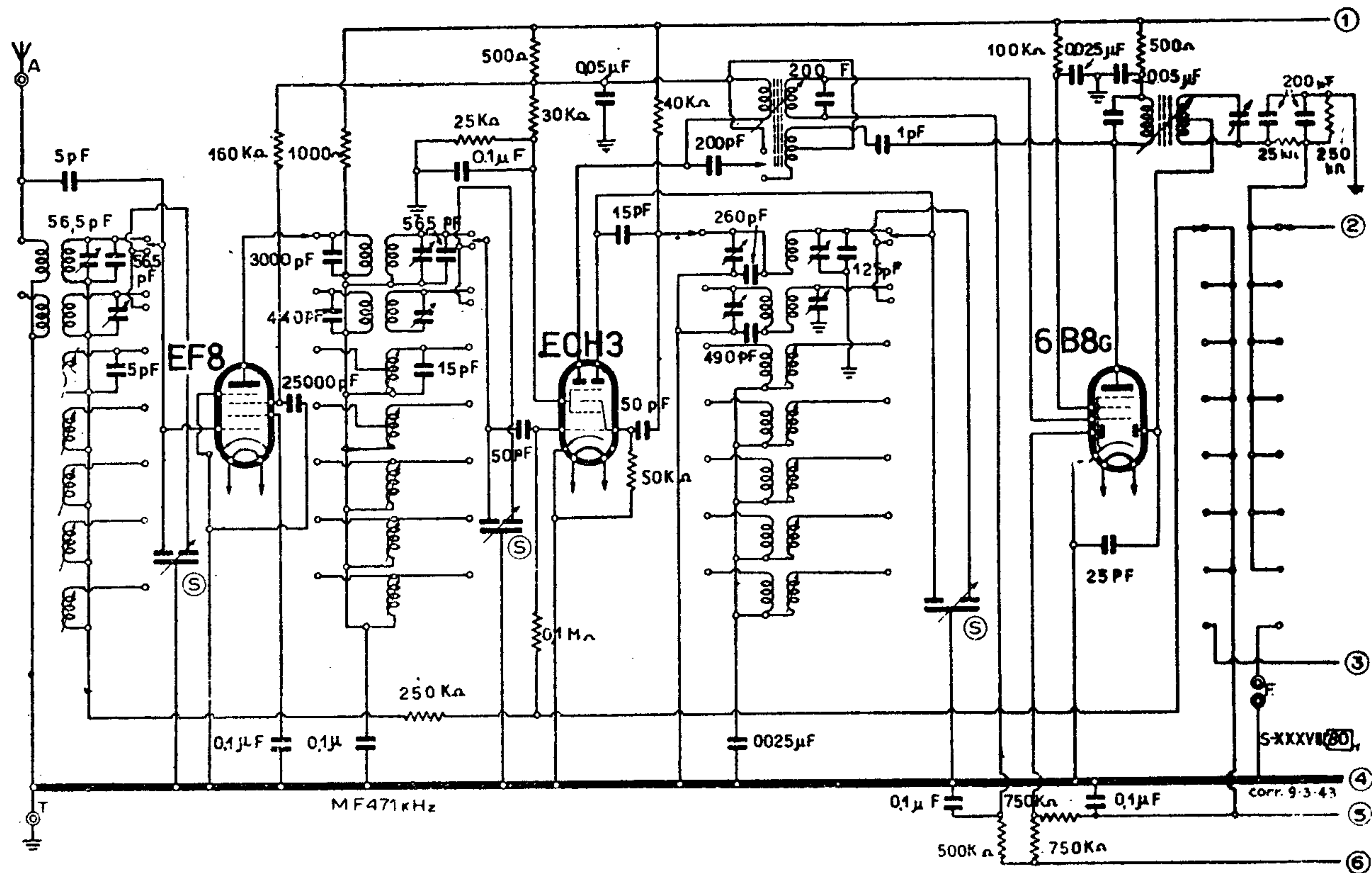
WATT RADIO - MOD. « MONDIALE » - PARTE AF - MF
