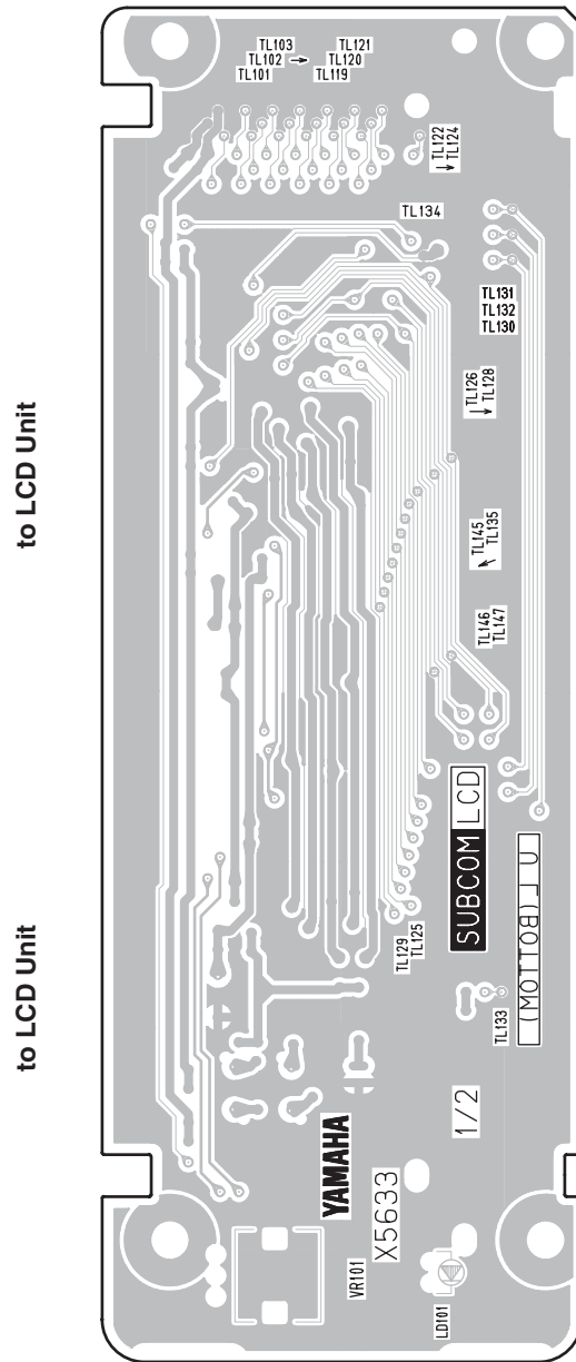
Pattern side (パターン側)
