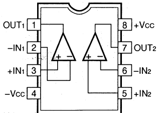
IC21, 22 : NJM2068D-D IC23, 24 : NJM5532D-D IC35 : BA15218 Dual OP-Amp
