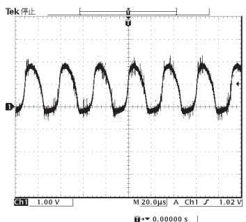
POINT ④ XL253 (Pin 11 of IC267)
