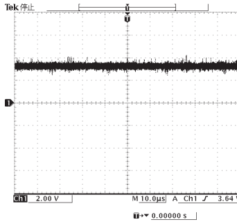
POINT (D) XL204 (Pin 11 of IC218)
