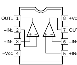
IC101, 210 : NJM2068D-D Dual OP-Amp
