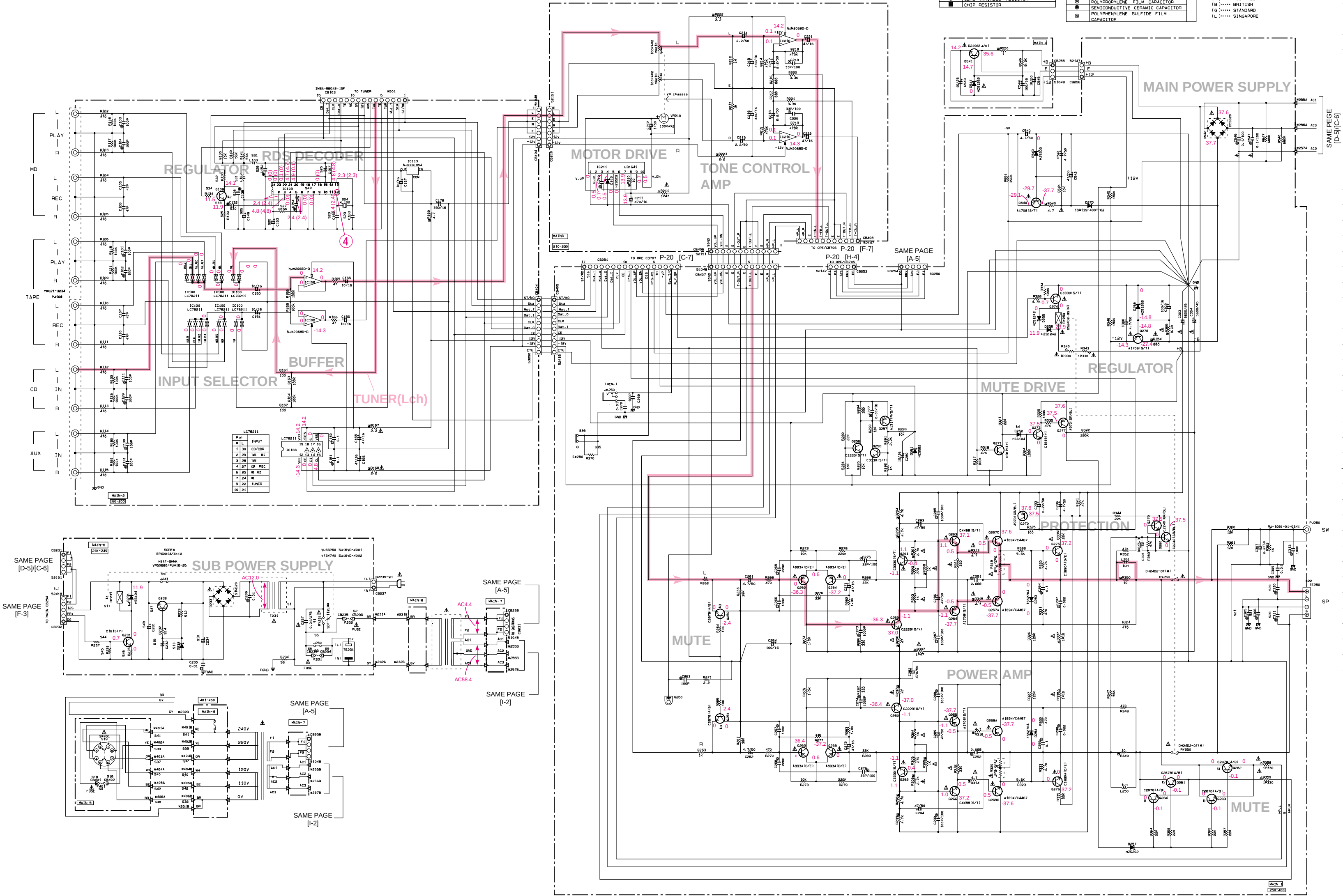
IC100 : LC78211 Analog Function Switch
