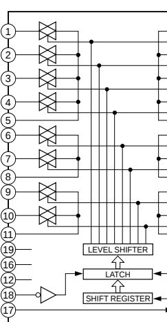
IC100 : LC78211 Analog Function Switch
