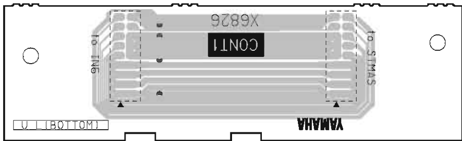
Pattern side (パターン側) 2NA-WF53540 ▲
