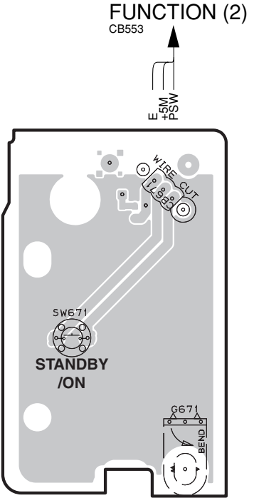
FUNCTION (5) P. C. B. (Side A)
