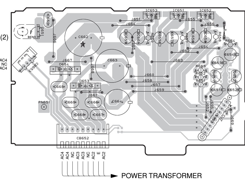
FUNCTION (4) P. C. B. (Side B)
