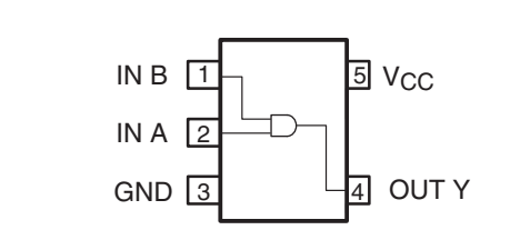
IC68: TC7SH08FU
