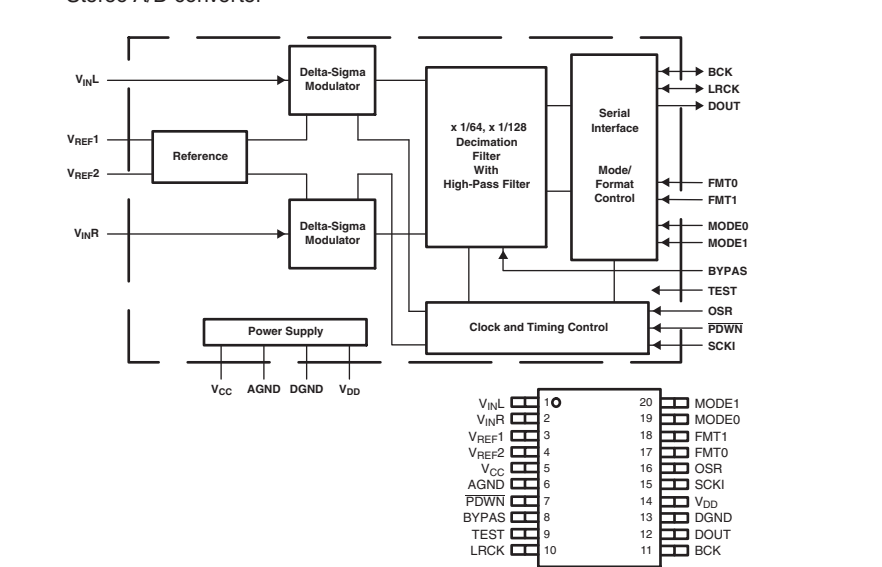
IC66: PCM1803DBR
