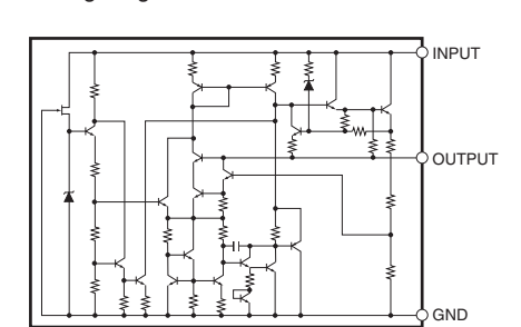
IC63: NJM78M05DL1A (TE1)
