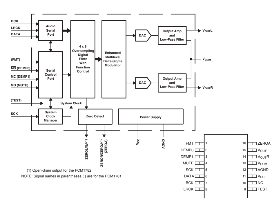
IC61: PCM1781DBOR
