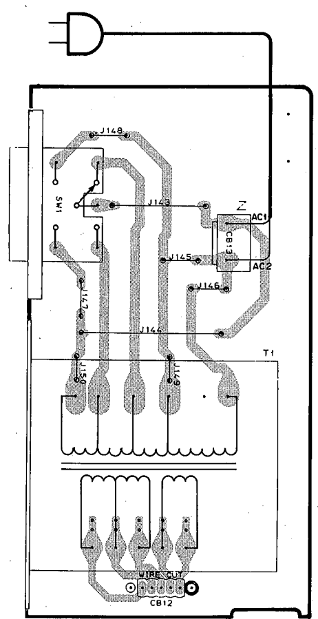
MAIN P. C. B. ( 4 )
