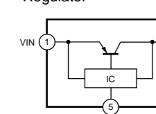
IC122: PQ018E201ZP Regulator
