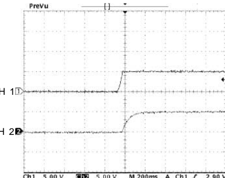
Point ④ (Pin 128 of IC901)
