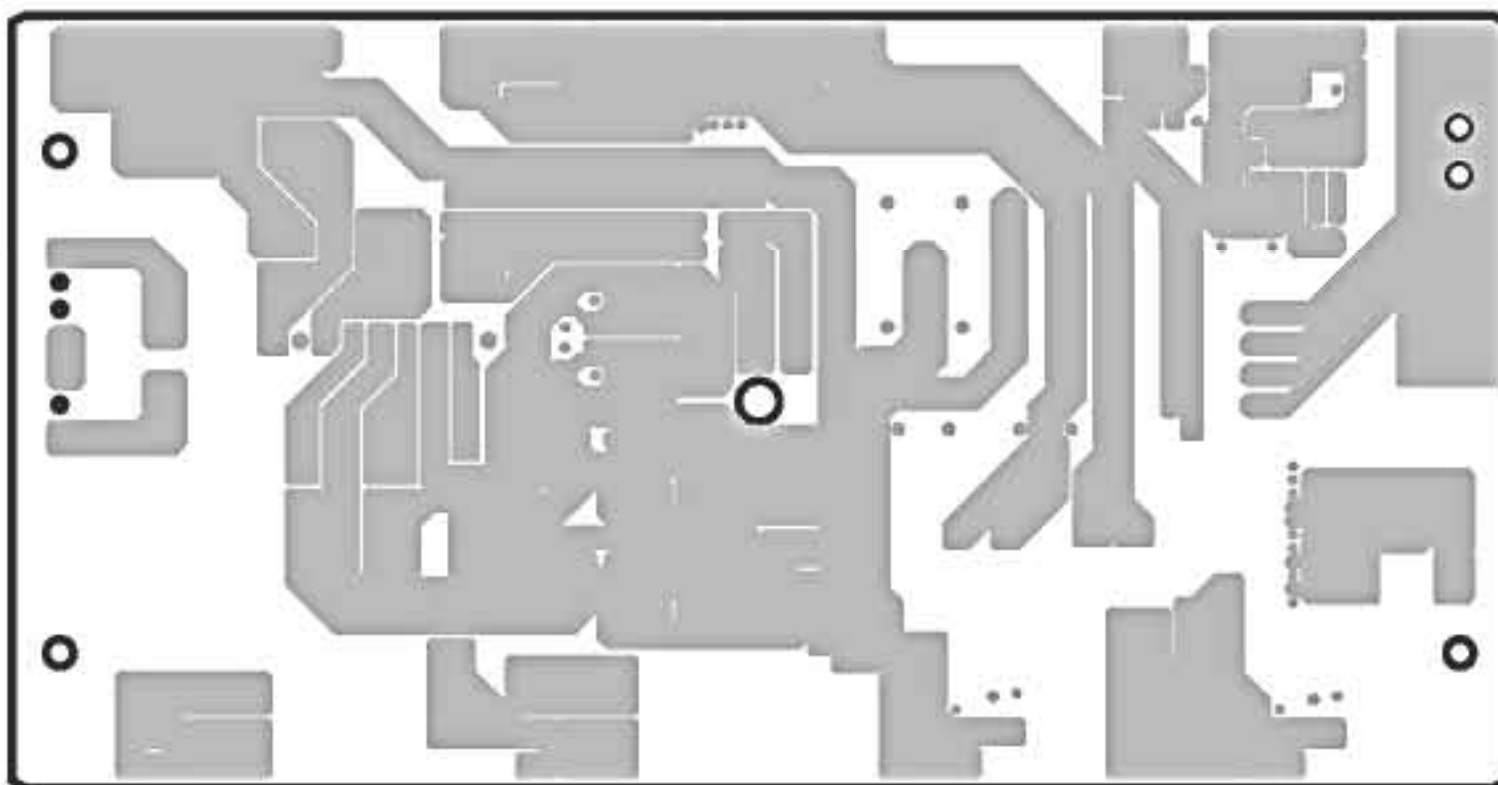
Pattern side (パターン側)
