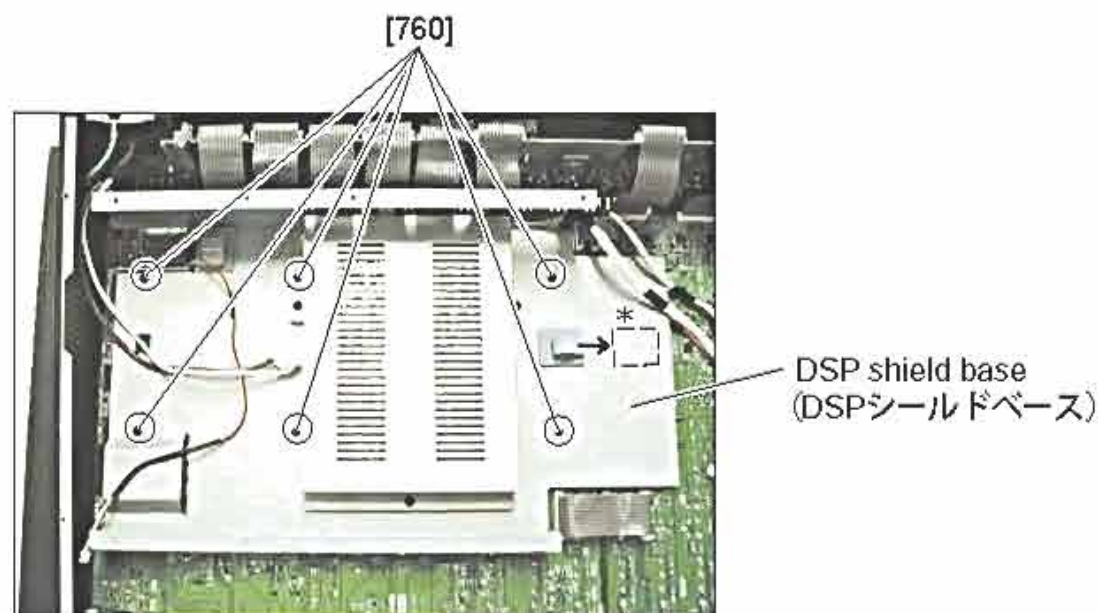
[760]: Bind Head Screw (+パインド小ネジ) 3.0X8 MFZN2Y (VD976600)
