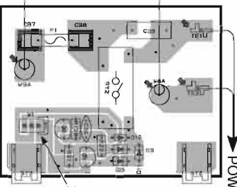
MAIN (2) P.C.B.
