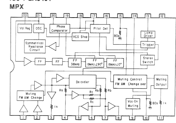
IC3 : LA3401
