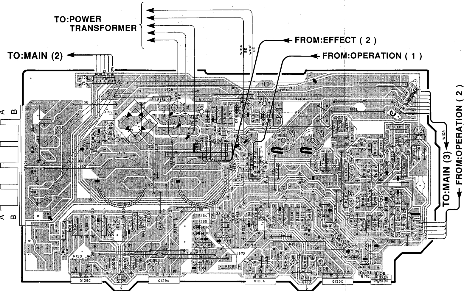
P.C.B. MAIN ( 1 )
