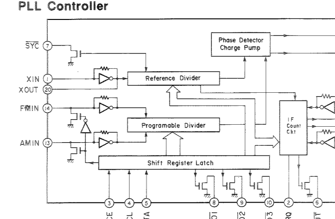
IC2 : LM7000N
