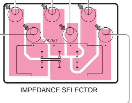
P. C. B. MAIN (8)
