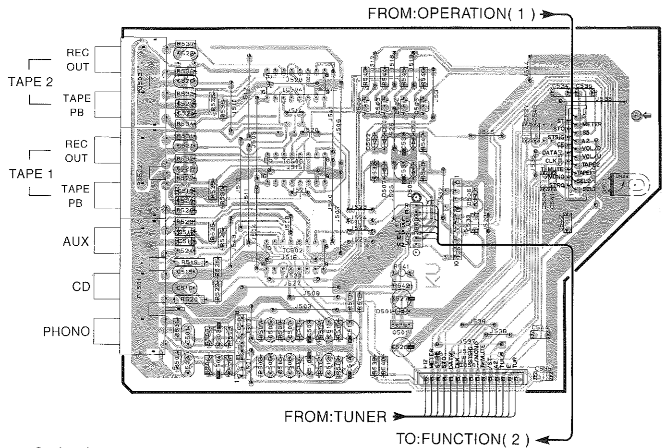
P.C.B. FUNCTION ( 1 )
