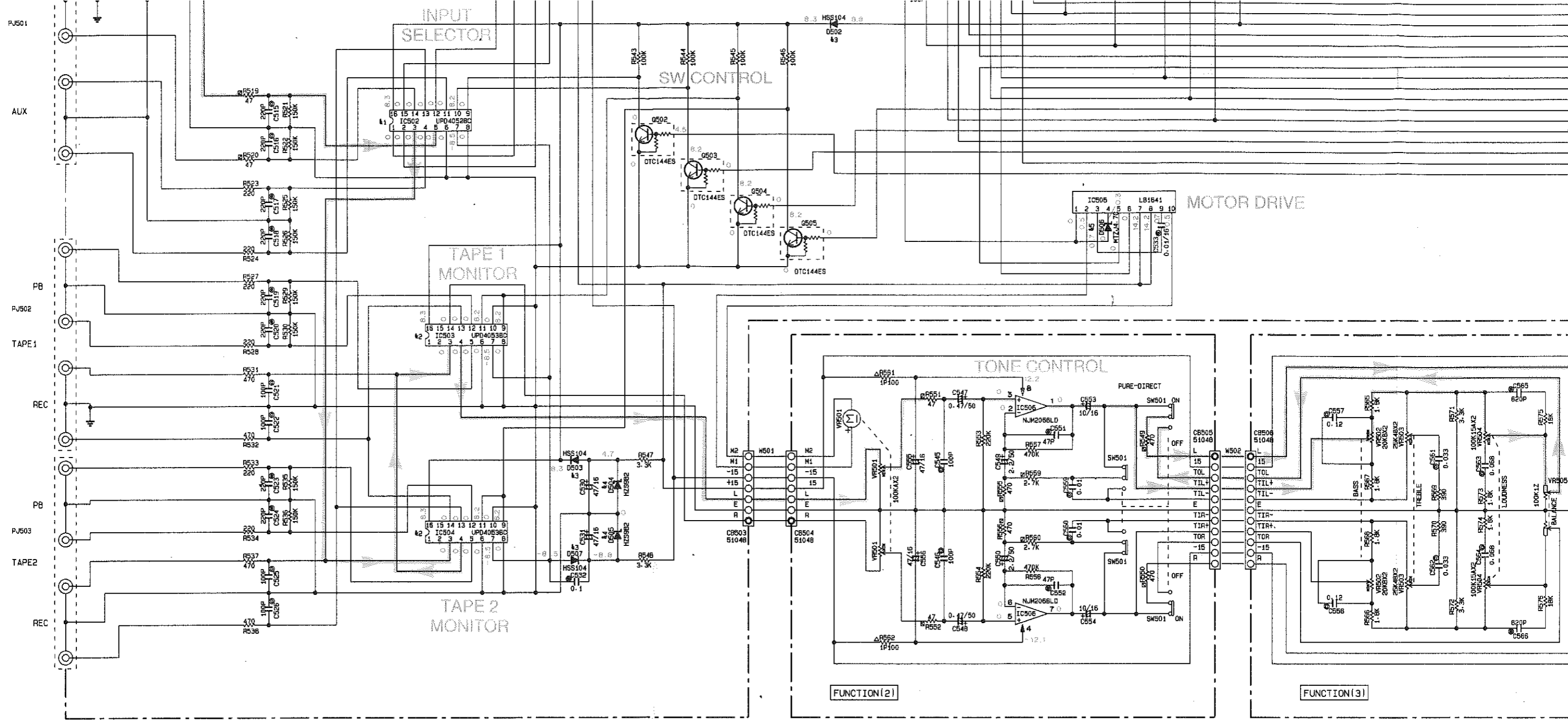
IC501, 506 : NJM2068L-D Dual OP-Amp
