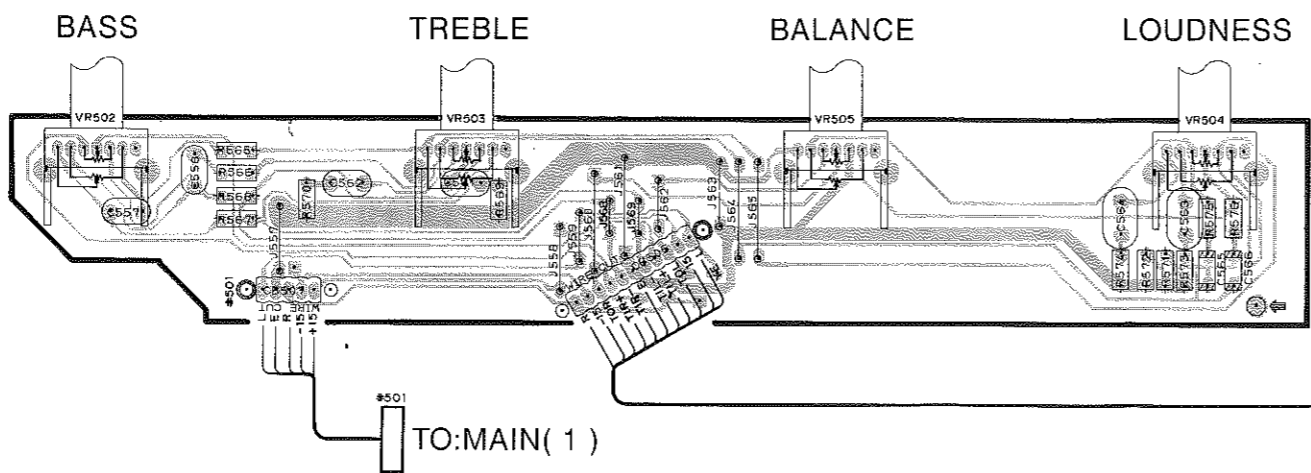
P.C.B. FUNCTION ( 3 )
