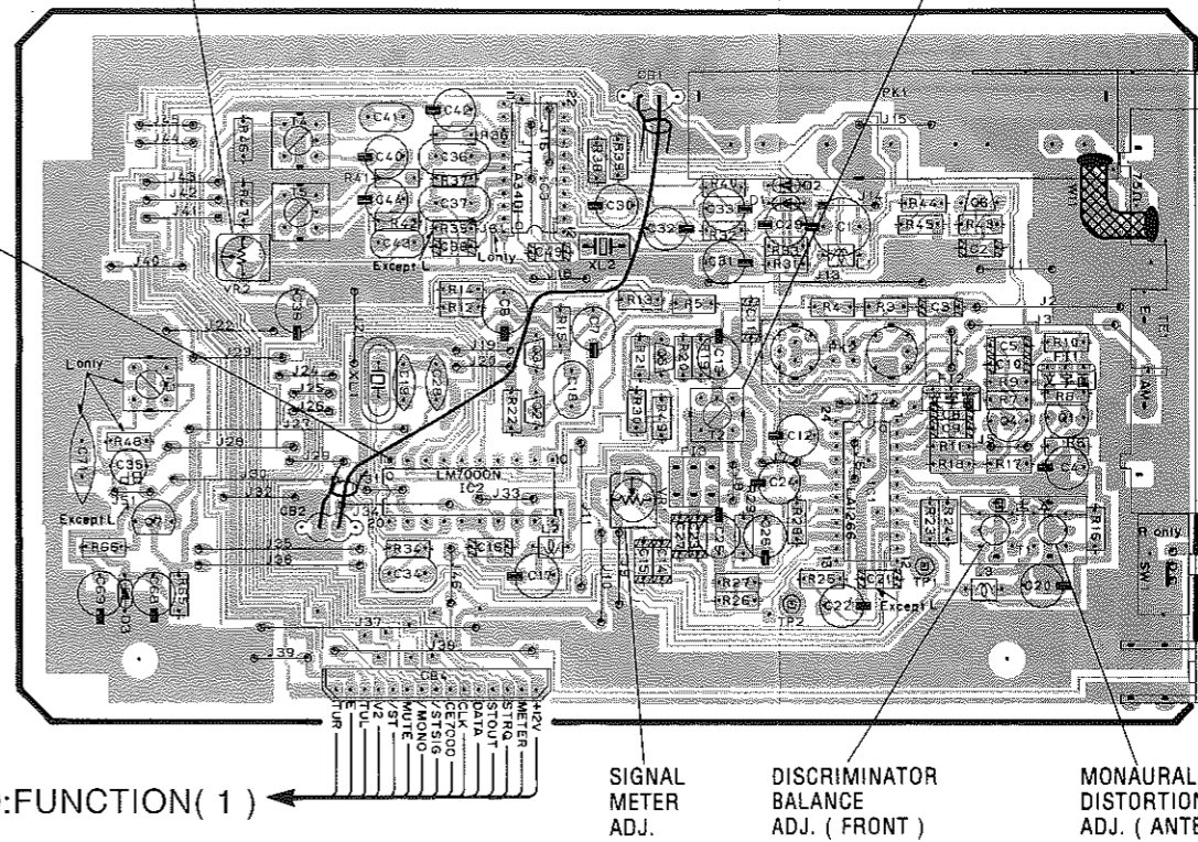
P.C.B. TUNER
