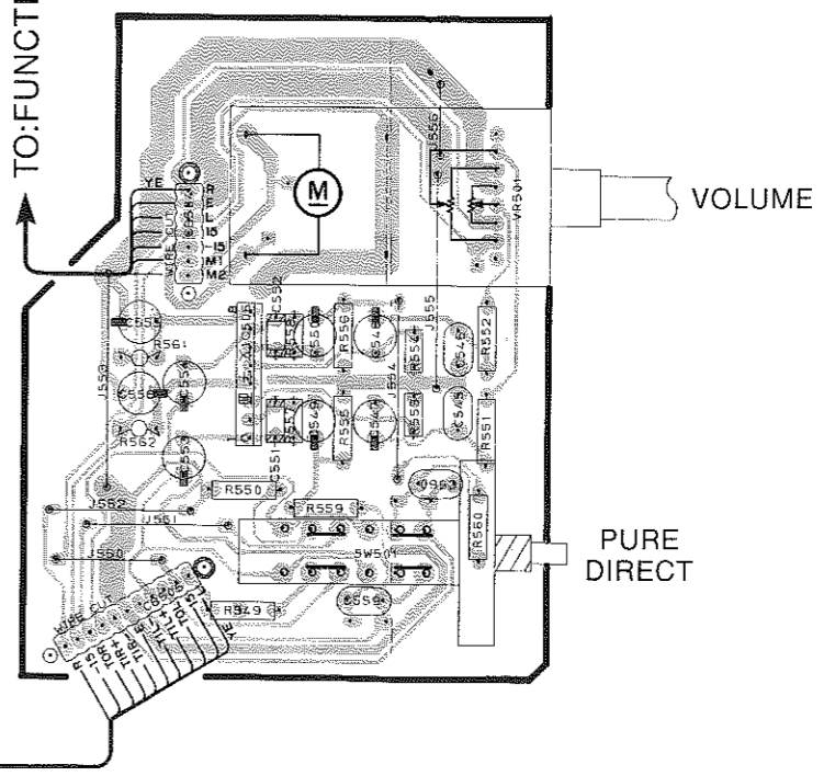
P.C.B. FUNCTION ( 2 )
