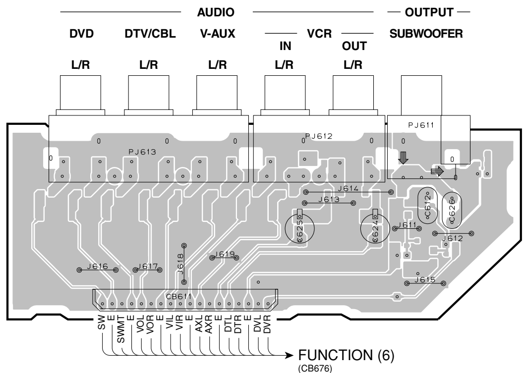
FUNCTION (3) P.C.B. (Side B)
