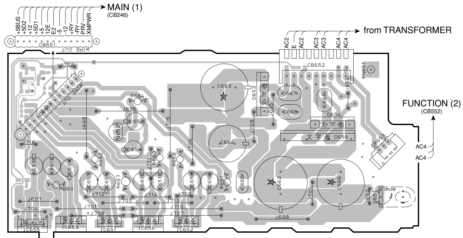
FUNCTION (4) P.C.B. (Side A)
