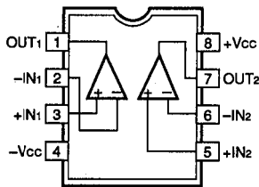
IC503, 507 : NJM2068D-D Dual OP-Amp
