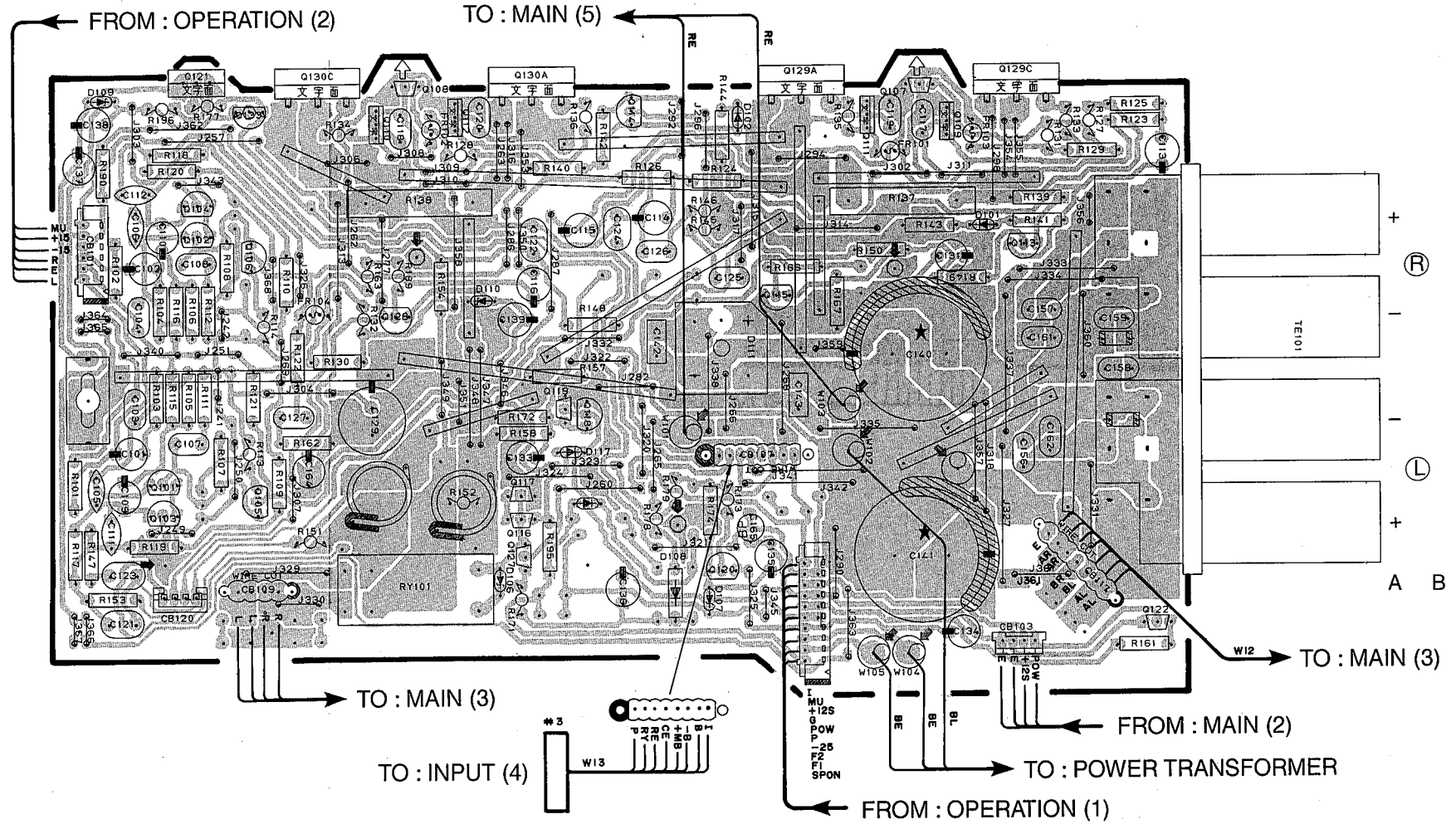
P.C.B. MAIN (1)
