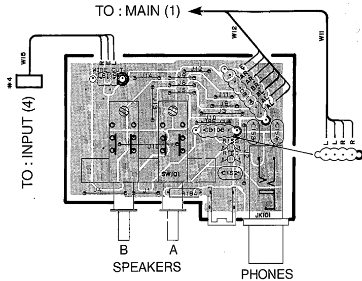
P.C.B. MAIN (3)
