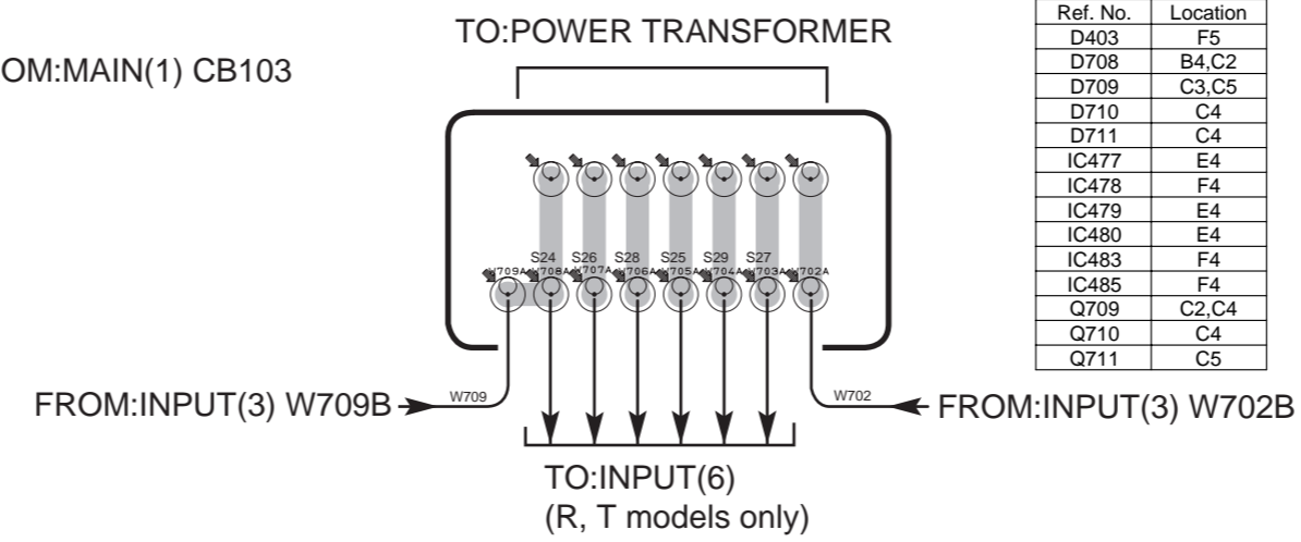
P.C.B INPUT (4)
