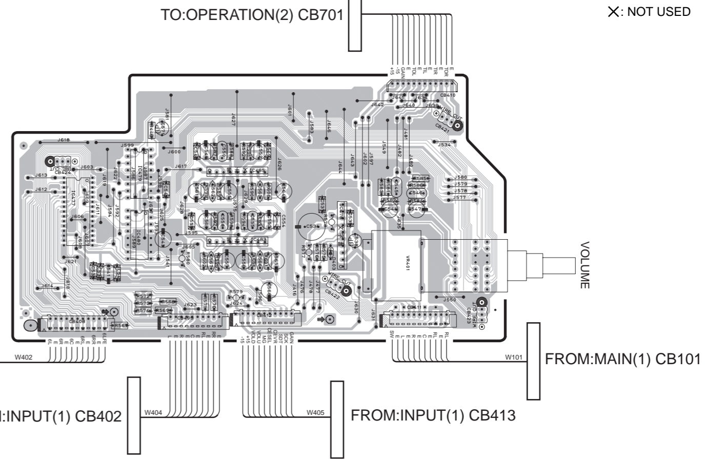
P.C.B INPUT (4)
