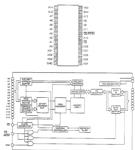
ICB : LM5P820-10 256K Pseudo Static RAM
