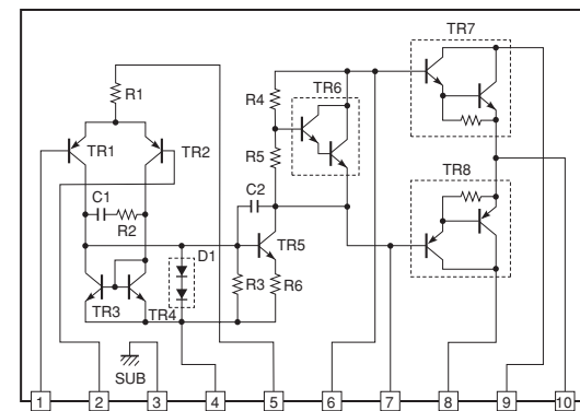
IC1: STK404-070 AF Power Amp
